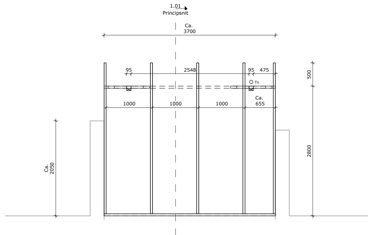
Stueplan - 1 : 50
